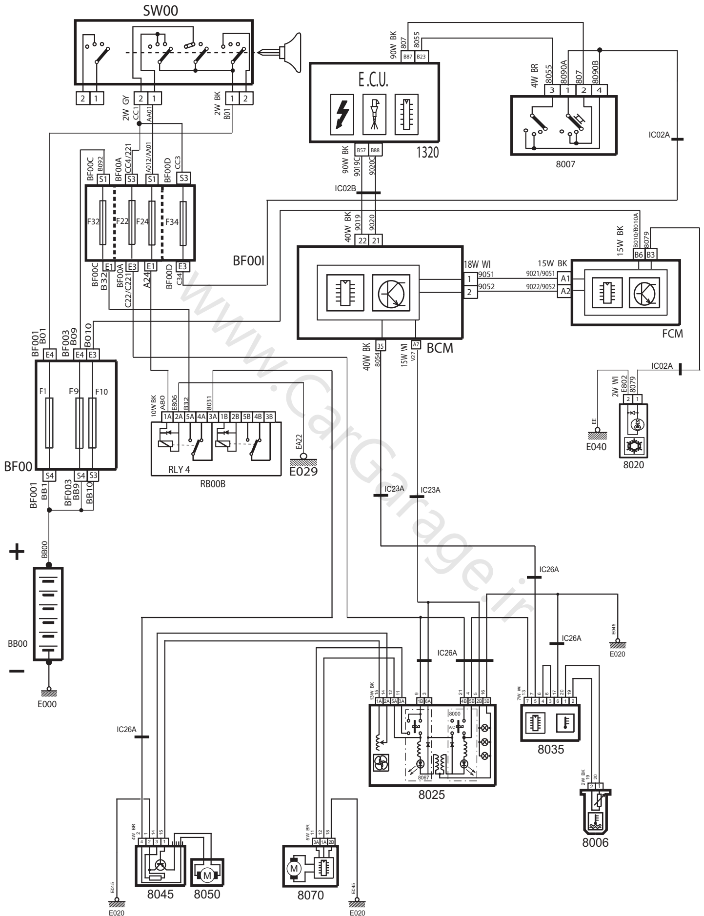
دیگرام شماتیک مدار سیستم تهویه مطبوع خودروی سمند با سیستم اکوماکس (ECO MUX) www.CarGarage.ir
